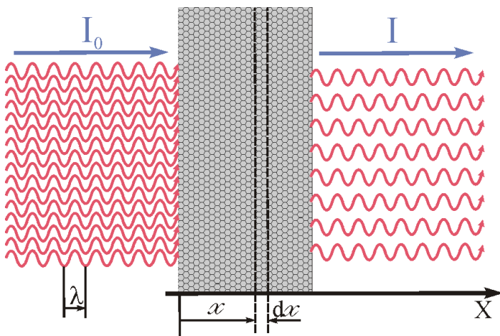
Fig. 1 Absorbția undelor mecanice în diverse medii.
